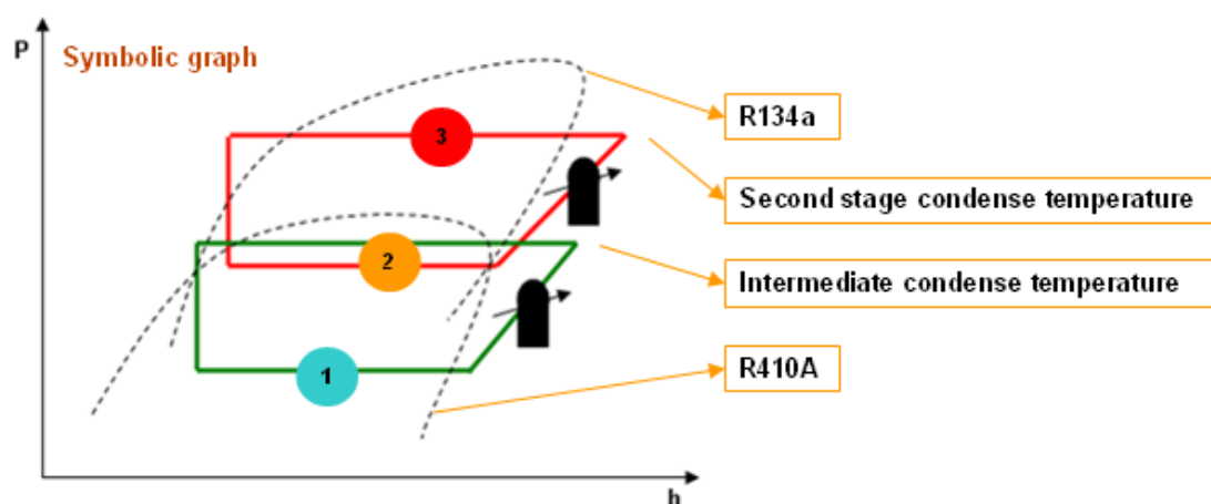
Διάγραμμα 3: Συμβολικό διάγραμμα Mollier cascade συστήματος
